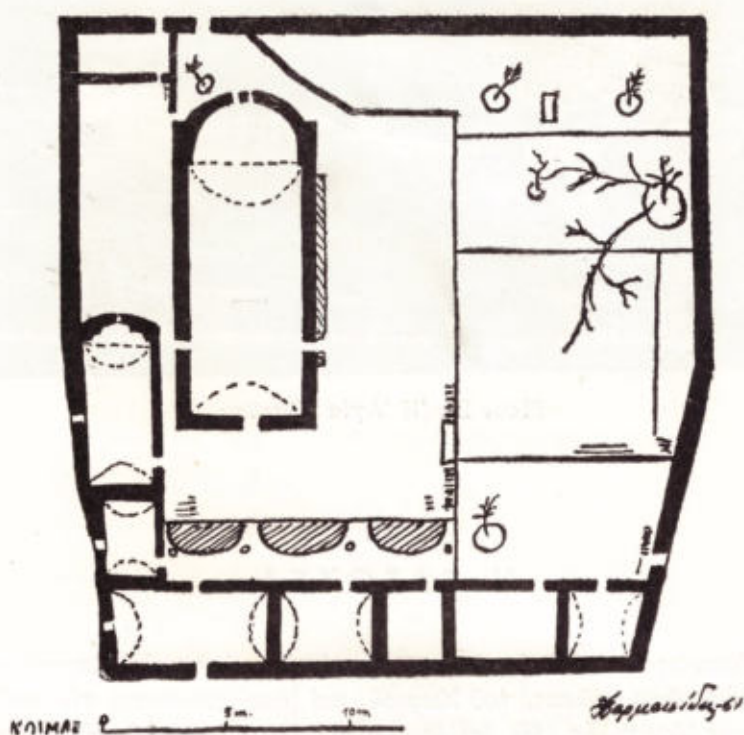
Εἰκὼν 21. Κάτοψις Μονῆς Ἑλεούσης
