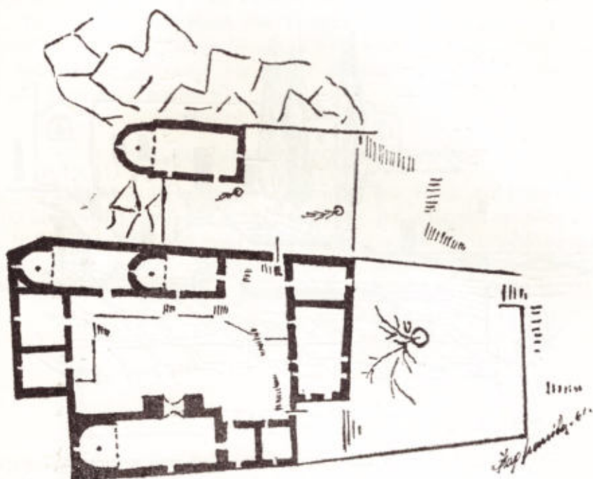
Εἰκὼν 3. Κάτοψις Μονῆς Προφήτου Ἑλίου
