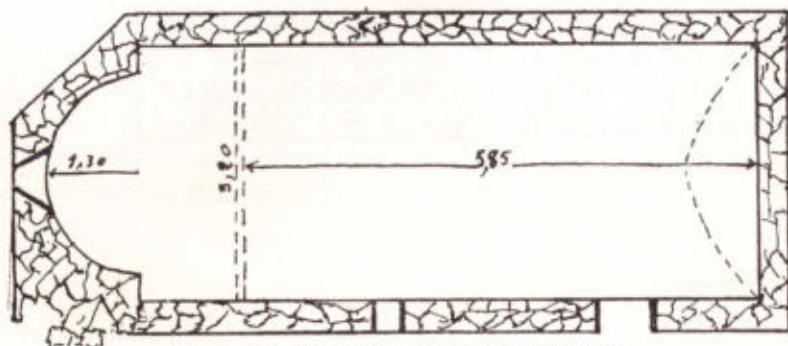
Εἰκὼν 15. Κάτοψις ναῖσκου Ὑπαπαντῆς.
