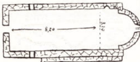
Εἰκὼν 25. Κάτοψις καθολικοῦ Ἑλεούσης
