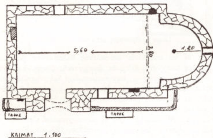
Εἰκὼν 5. Κάτοψις ναοῦ Προφήτου Ἡλίου
